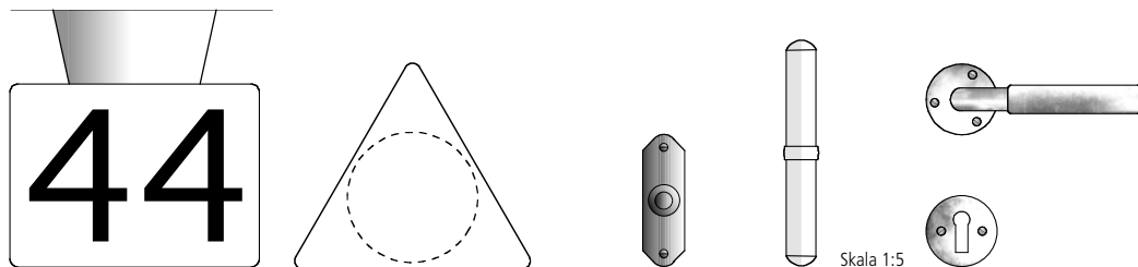
Utomhusarmatur med trekantig kupa av opalglas med gatunummer. Ringklocka av svartlackad plåt. Gångjärn med ny design. Dörrtrycke med slät rosett och nyckelskylt av förnicklad mässing.
